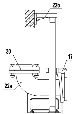
Установка на автоматическую трубную муфту (Z)
