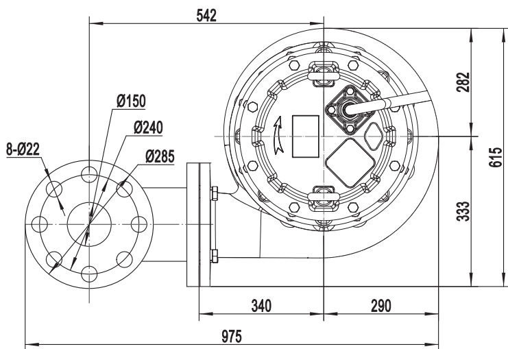
Установка со съёмным жестким трубопроводом (У)
