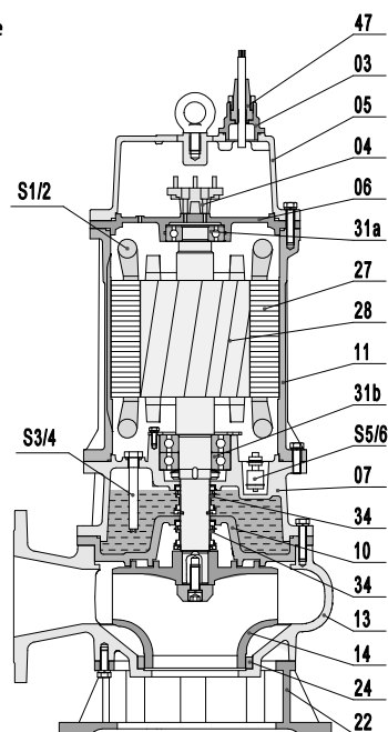
Свободстоящее исполнение под жесткий трубопровод (Y)
