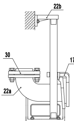
Установка на автоматическую трубную муфту (Z)
