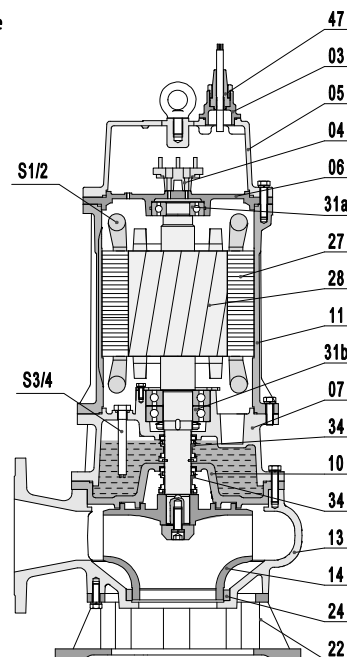
Свободностоящее исполнение под жесткий трубопровод (Y)
